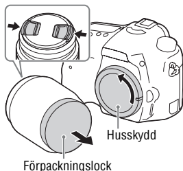
Främre linsskydd
