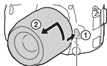
Botón de liberación del objetivo
