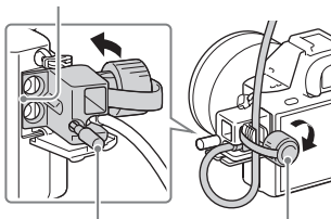
Befestigungsschraube Befestigungsknopf
