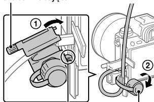
Śruba mocująca
