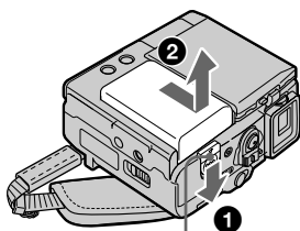
BATT release lever / Manette de relâche BATT
