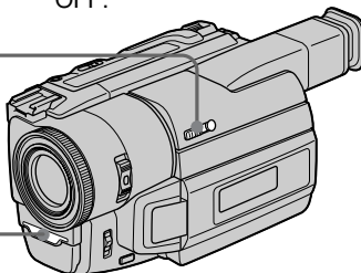
NightShot Light emitter/ Излучатель подсветки для ночной съемки
