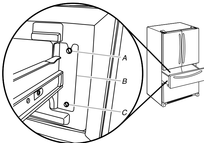
A. Afloje los tornillos de la parte superior B. Soporte de la guía del cajón
