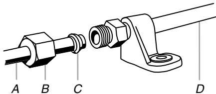
A. Línea de agua de la casa C. Férula (adquirida) B. Tuerca (adquirida) D. Tubería de agua del refrigerador
