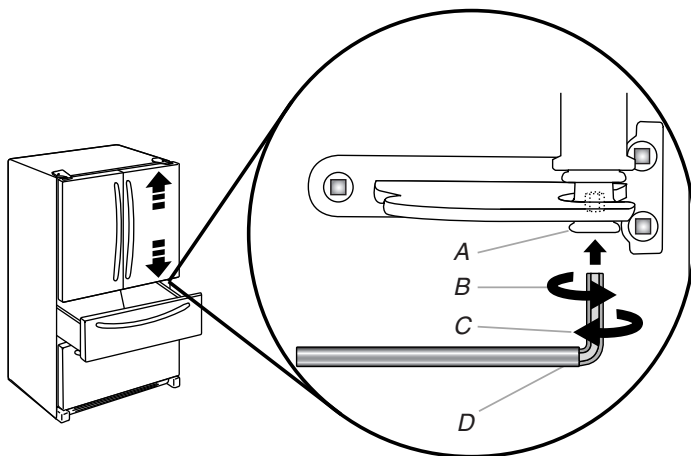
A. Pasador de la bisagra inferior B. Gire hacia la derecha para levantar C. Gire hacia la izquierda para bajar D. Llave hexagonal en L de \frac{1}{8} "
